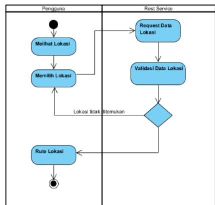
Gambar 2.7 Activity Diagram Pengguna Android
