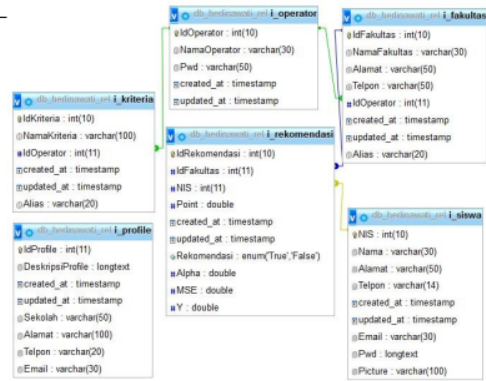
Gambar 2.3 Relasi Tabel
