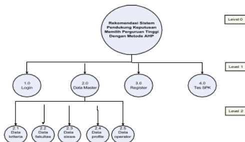
Gambar 2.7 Bagan Berjenjang
