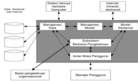
Gambar 1.1 Komponen SPK
