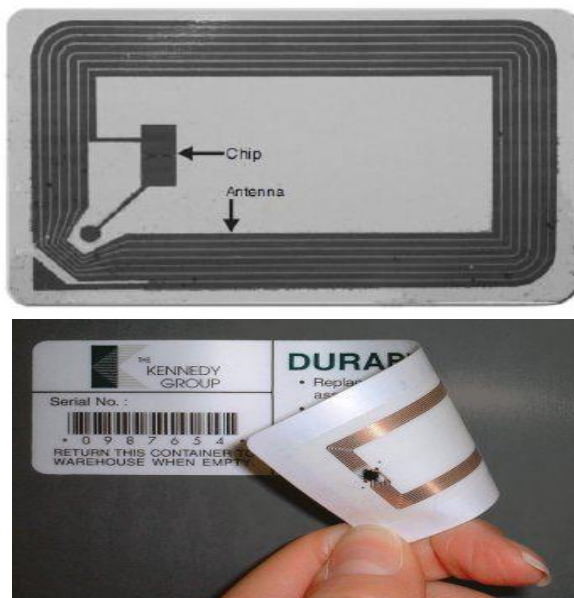
Gambar 2. Tag RFID
