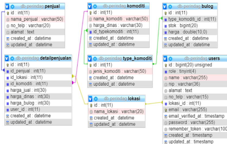
Gamabar 1. Desain Relasi Database
