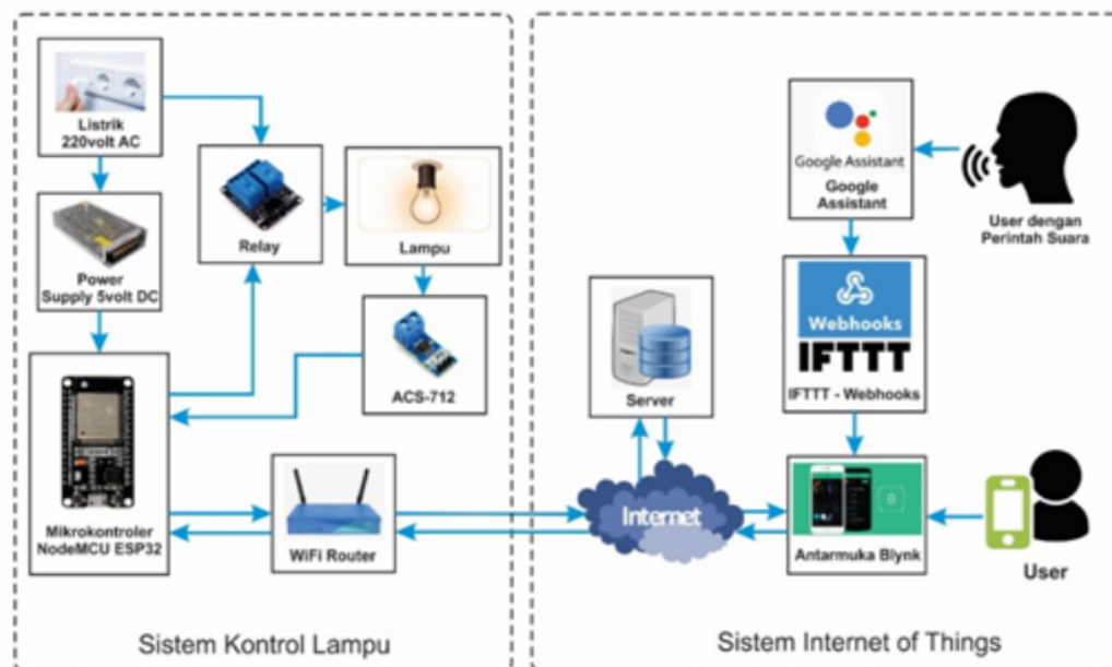
Gambar 2. Diagram blok sistem kontrol lampu berbasis IoT
