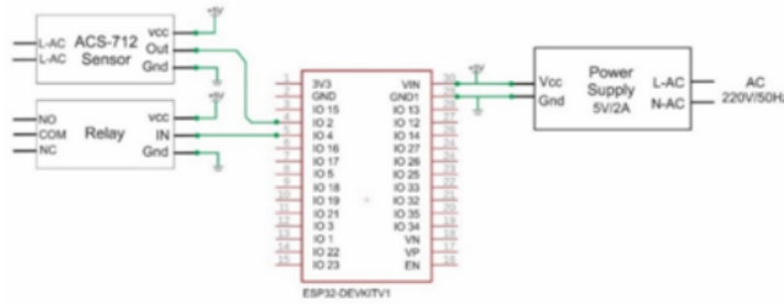
Gambar 3. Skematik rangkaian sistem kontrol lampu
