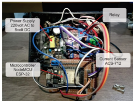
Gambar 8. Rangkaian perangkat keras
