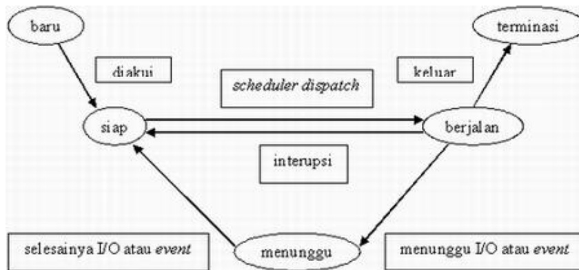
Gambar 4.1. Keadaan Proses.
